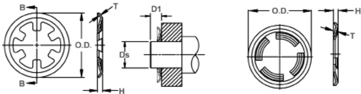
外径 B-B 横断面图
