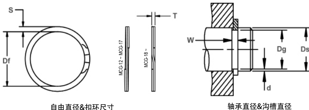
自由直径&扣环尺寸
