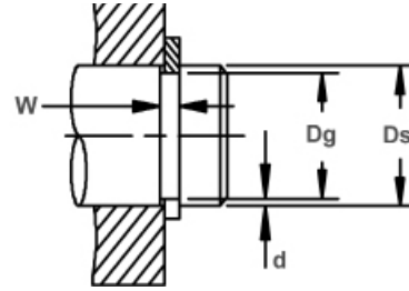
轴承直径&沟槽直径
