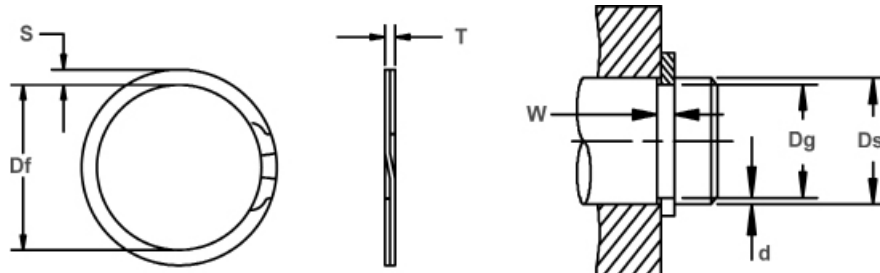
自由直径&扣环尺寸
