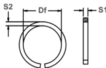
自由直径&扣环尺寸
