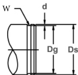
轴承直径&沟槽尺寸
